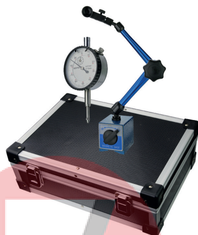
01005025: Messuhr (Nr. 01023005) und Stativ (Nr. 06071009) im Alukoffer 31,5 x 22 x 11,5 cm / in aluminium case
